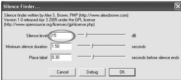
Abbildung 12: Silence Finder
